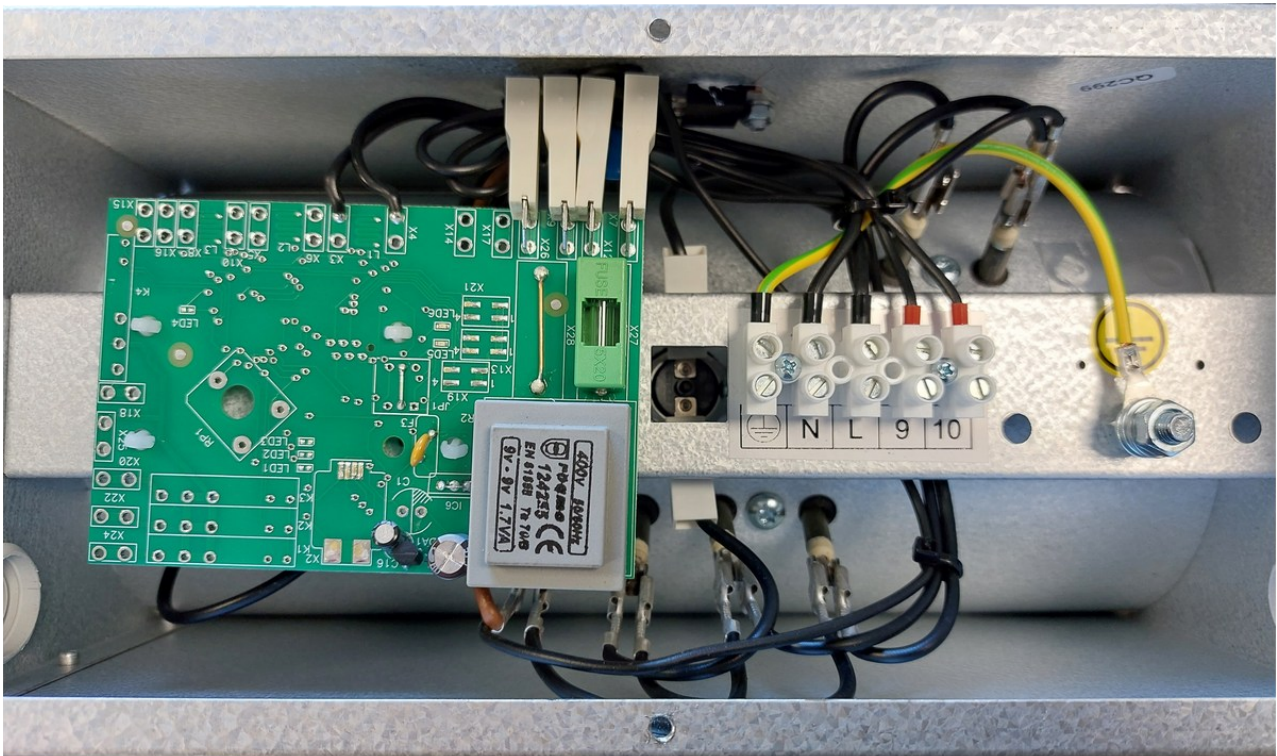
230VAC-1ph met 0-10V ingang (klem 9 en 10)
