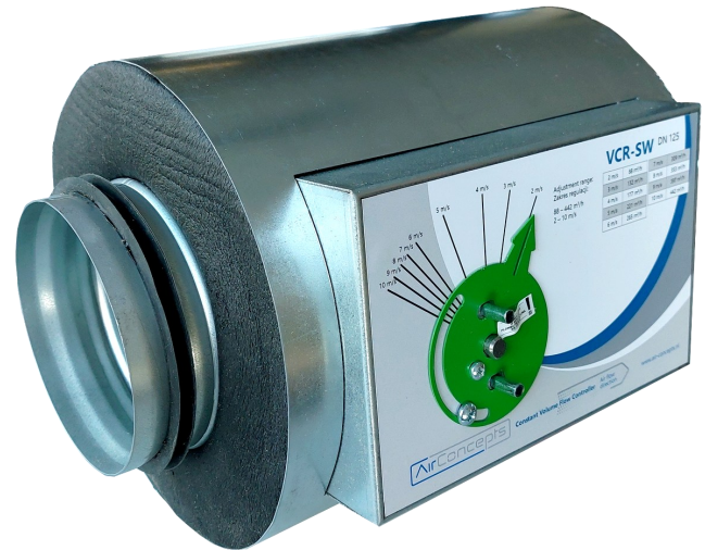
VCR-DW-125 (dubbelwandig)
