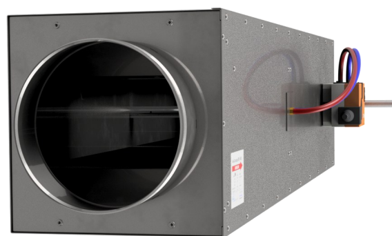
VSR-QAR-BE1 (retour unit met Belimo LMV-D3-MP regelaar)
