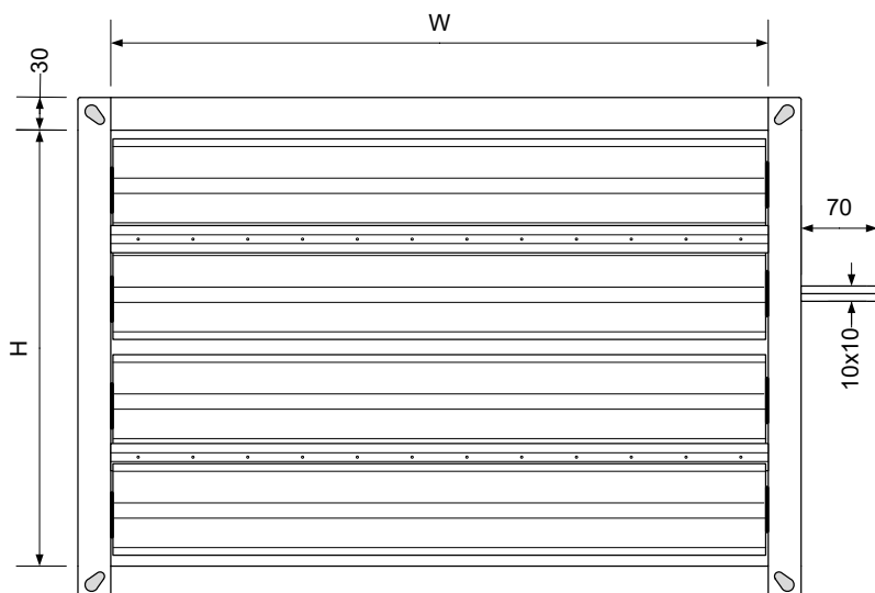
Type VSQ-SW (enkelwandig), model 600x400
